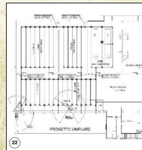
22 Progetto in unifilare per impianto di macellazione carni rosse
