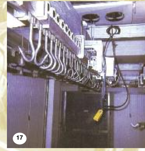
17 Tratto con divaricatore per carni
