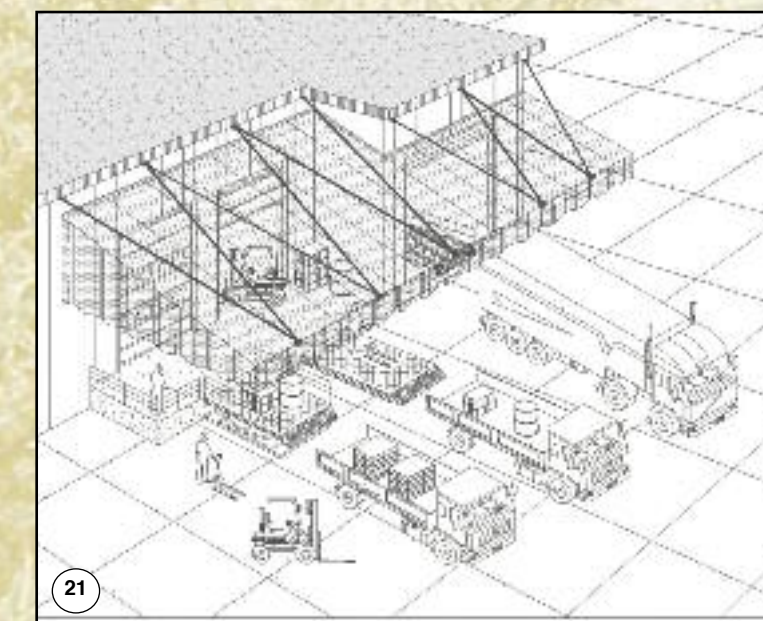
21 Panoramica di uno scarico merci con copertura a sbalzo
